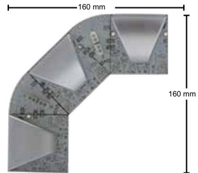
5-53123: 3 módulos ILS de 3 LED y 9 W con 2 conectores de alimentación de enlace en ángulo 5-50002
